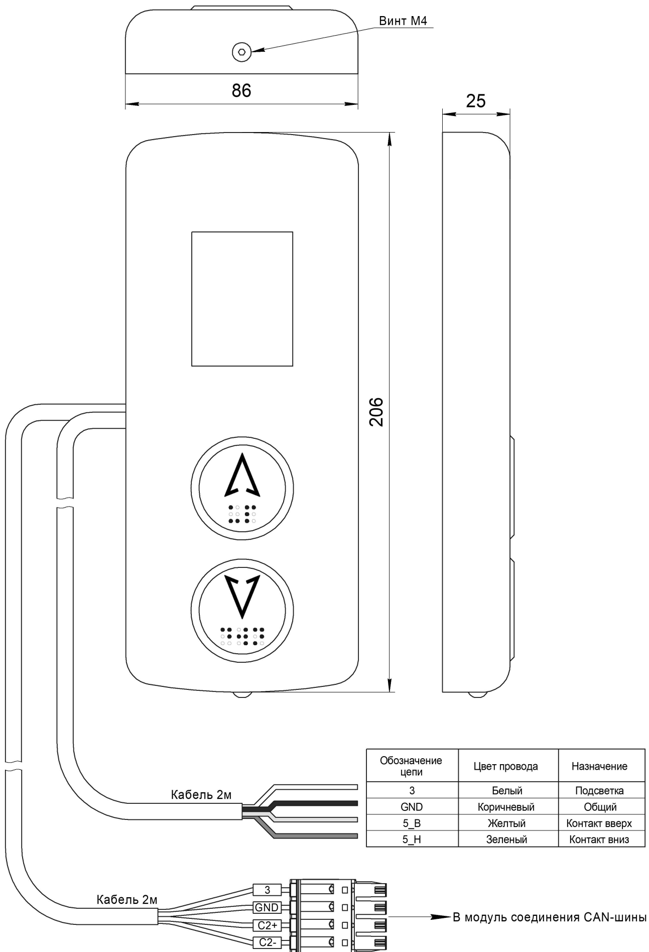
Рис.1 Внешний вид, габаритные и установочные размеры Вызывного поста ВП-2103-1086-08
